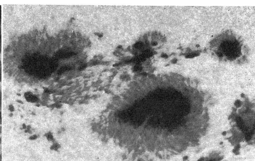
\overline{20} (f) 01 27 04 UT OCT.13
