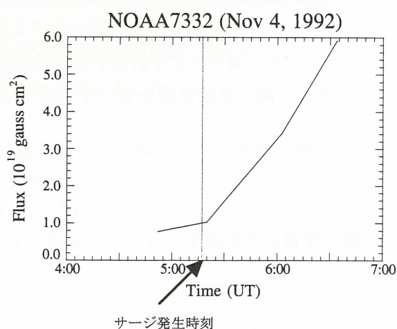
図3. 孤立磁場領域の磁場強度の時間変化の様子
