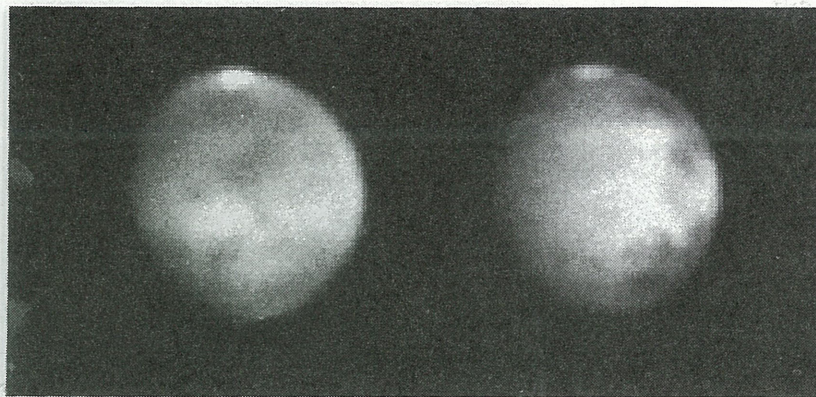
図3. 左：火星タルシス地方の朝雲（中央少し左よりの大きな明るい斑点。120 W, 10 N）。その雲の縁にある複数の暗い斑点は火山の峰である。（Apr. 13, 1994. CM=112, Ls=84）。右：ほぼ同時刻の赤色光による像。雲を透して地面の様様が見えている。CM：中央経度。Ls：火心太陽黄経。
