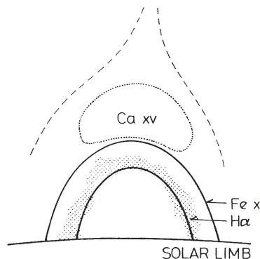
a：コロナの微細ループ構造：左の黒い小山がフレアループ。 b：フレアループの温度構造
