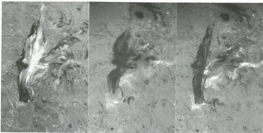
b：噴出フィラメントの速度場
