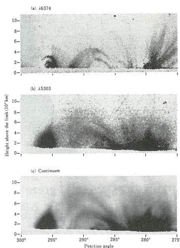
a：コロナの微細ループ構造：左の黒い小山がフレアループ。 b：フレアループの温度構造
