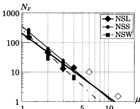
図 5 \mu - N_F 関係
