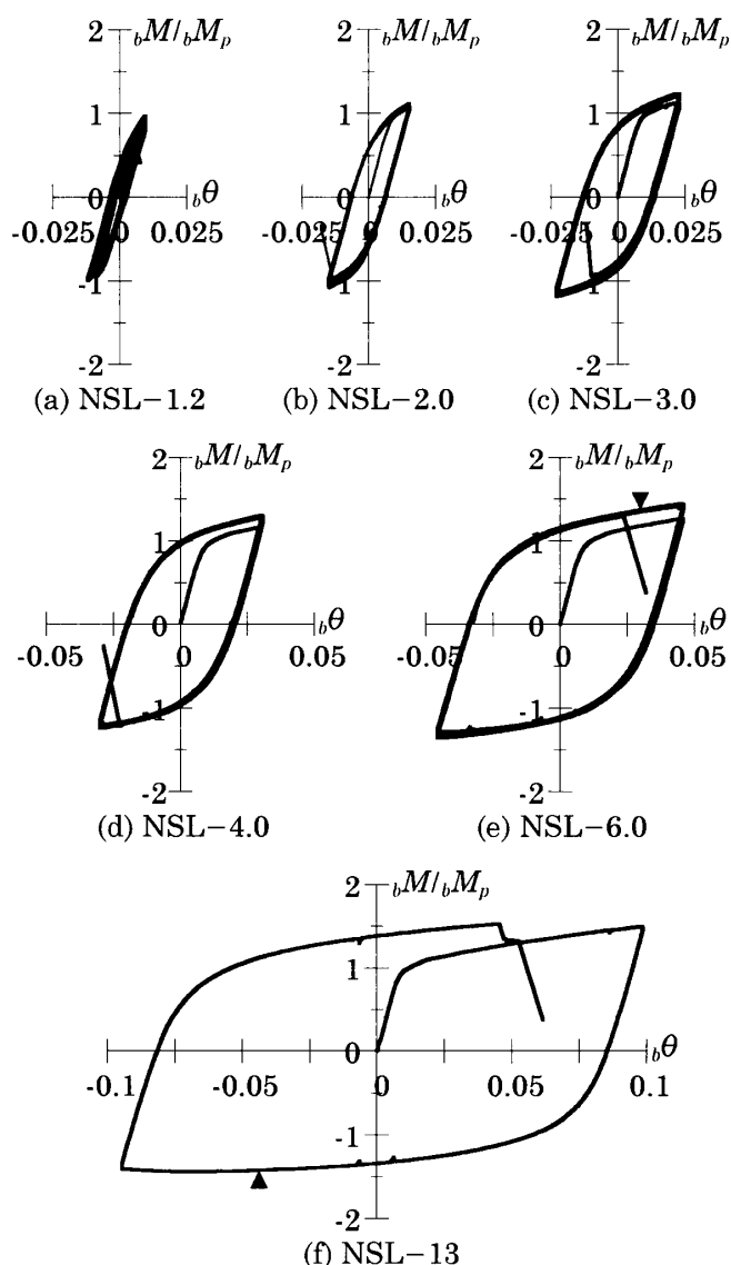
図3 各実験の履歴曲線
