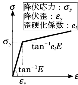
図12 応力-歪関係
