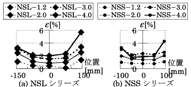
図13 実験で計測された歪
