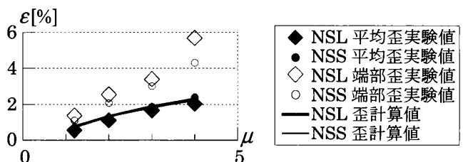
図14 歪の比較
