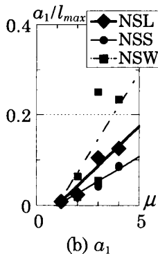
図 9 亀裂速度の係数
