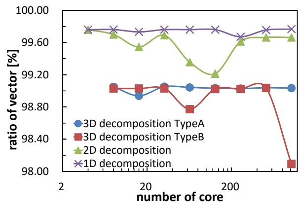
図 3 MHD コードのベクトル化率
