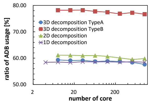
図 4 MHD コードの ADB 利用率
