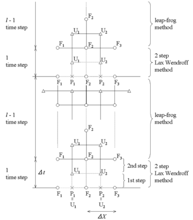
図 1 Modified Leap Frog 法の計算スキーム
