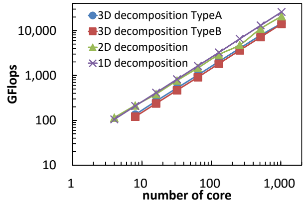
図 2 SX-ACE での MHD コードの性能
