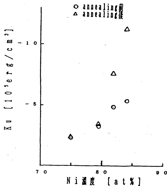
図2 Kuの組成依存性
