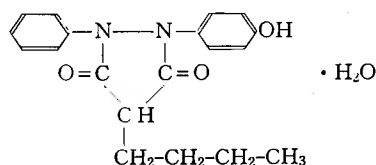
1-phenyl-2-(p-hydroxyphenyl)-3,5-dioxo-4-n-butylpyrazolidine monohydrate
