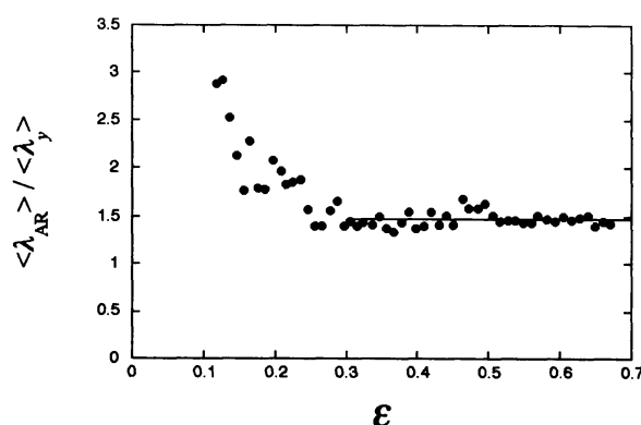
図12 図9における \langle \lambda_{AR} \rangle と欠陥の方向の間隔の平均 \langle \lambda_y \rangle の比. 欠陥格子が形成される \varepsilon \geq 0.3 では、比が一定に保たれる。
