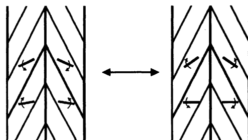
図16 振動している欠陥格子における director の回転. abnormal rollsの finestructureの明るさの振動(図16(b))と, 像の明るさとCの回転の関係(図6(b))とを対応させることによって推測される directorの回転の様子を, 模式的に表しており, 左図と右図の間で時間的に振動する.
