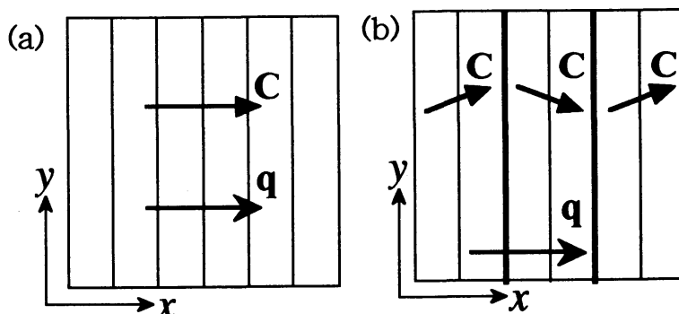
図4 対流の波数ベクトル \mathbf{q} と director \mathbf{C} 。
