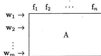
図 1: データ行列 A の構成
