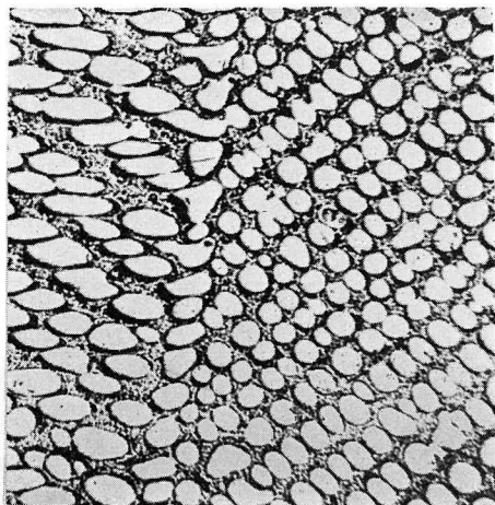
Fig. 7. ×150 24 wt. % Au, air-cooled ( \text{AuPb}_2 +eutectic)
