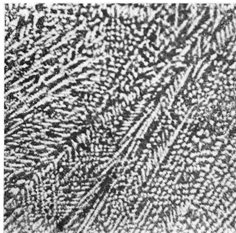
Fig. 6. ×150 24 wt. % Au, quenched ( \text{AuPb}_2 +eutectic)
