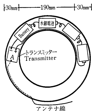
第 1 図 発信器をつけた首輪
