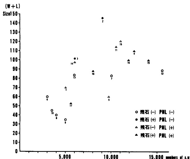
Fig. 3. 結石の長径と短径の和との衝撃波数.
