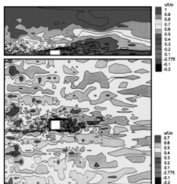
人工的に生成した流入乱流場を用いた角柱周りの非定常流れ場の数値計算
