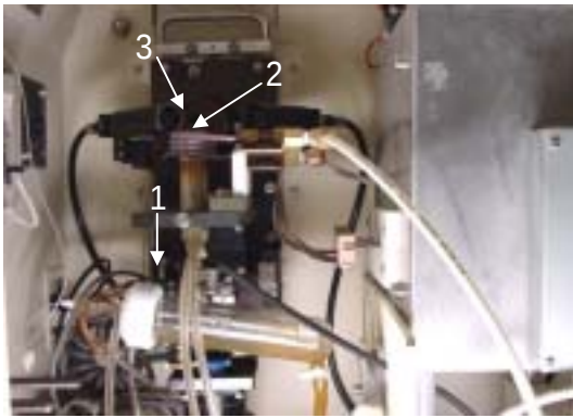
写真：地盤環境影響物質の微量分析装置；(左)高周波プラズマ発光分析装置による分析。ネブライザ、チェンバ1)より霧化した試料をプラズマ2)内へ導入する。高周波融合プラズマによって試料に電気/熱エネルギーを与えることにより発光させ、放射された光を3)を通して内部の分光器により各元素固有のスペクトル線に分け、スペクトル線の有無と強度から試料中の元素の定性/定量分析を行う。無機汚染物質に適用。(右)ガスクロマトグラフ質量分析計。有機系汚染物質の定性/定量分析に適用。
