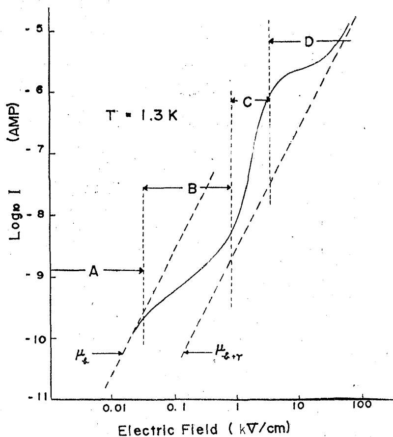
Fig. 2 IV-特性
