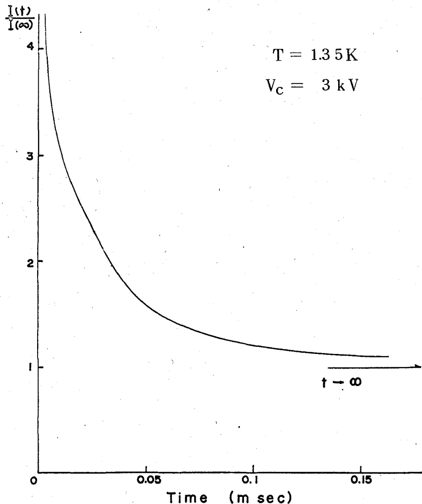
Fig. 8 I(t) の計算
