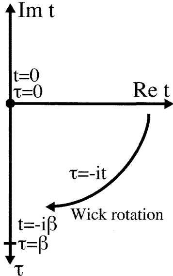
図8 Wick 回転
