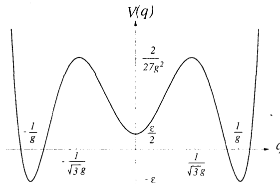
図 1: 式 (1) で与えられるポテンシャルの形状
