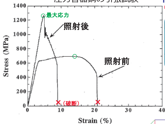
圧力容器鋼の引張試験
