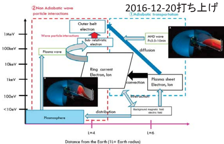
外部供給説と内部加速説の概略図
