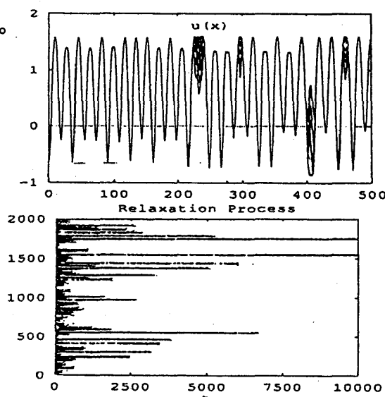
図 1: ある dynamical glass のアトラクター。時間的には 4 ステップ後にこのパターンに戻る。空間パターンの凹凸には周期性は見えず、異なった初期条件からは異なった凹凸のパターンに落ち着く。
