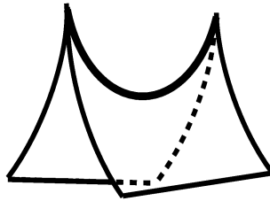
cuspidal edge
