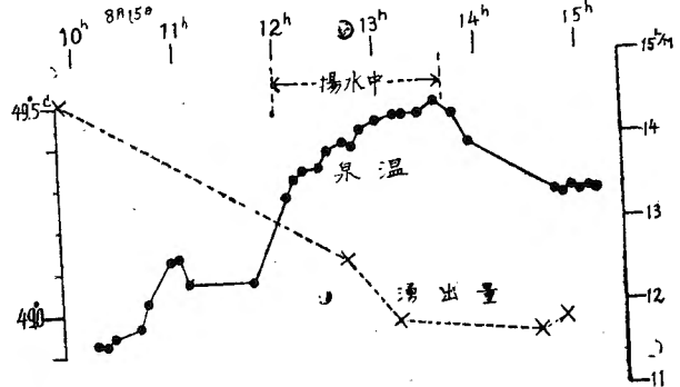
第4圖 亀No. 318.1の揚水中のNo. 318の泉温湧出量の變化
