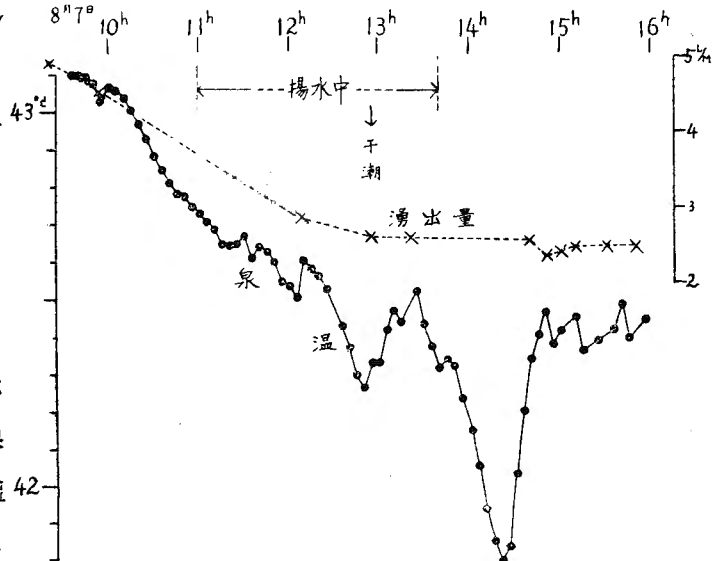
第7圖 別, No. 19の揚水中に於ける, No. 32の泉温湧出量の變化
