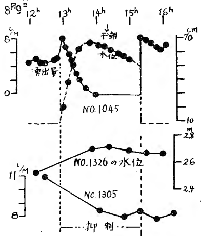
第11圖 A 別No.104の湧出抑制による周邊温泉の影響
