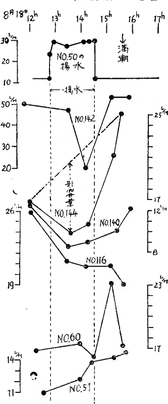
第12圖 A 龜 No.50の揚水による周囲温泉への影響
