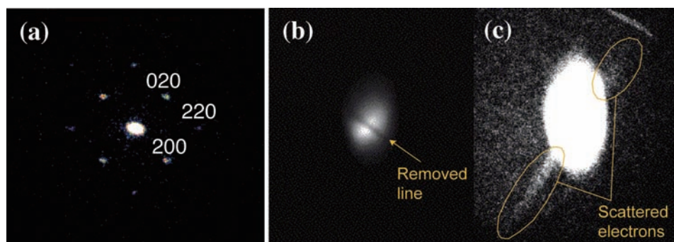
(a) 超高強度短パルスレーザー生成プラズマ電子を 500 fs に圧縮し、この電子パルスにより撮像した金の単結晶薄膜の電子線回折像。電子パルス幅測定法として電子ビームと超短パルスレーザーとの相互作用相関測定法も実証した。 (b) 電子ビームの一部がレーザーの光圧により散乱され線上に除去されている様子が見られる。 (c) レーザービームと直交する方向に散乱している電子が観察された。
