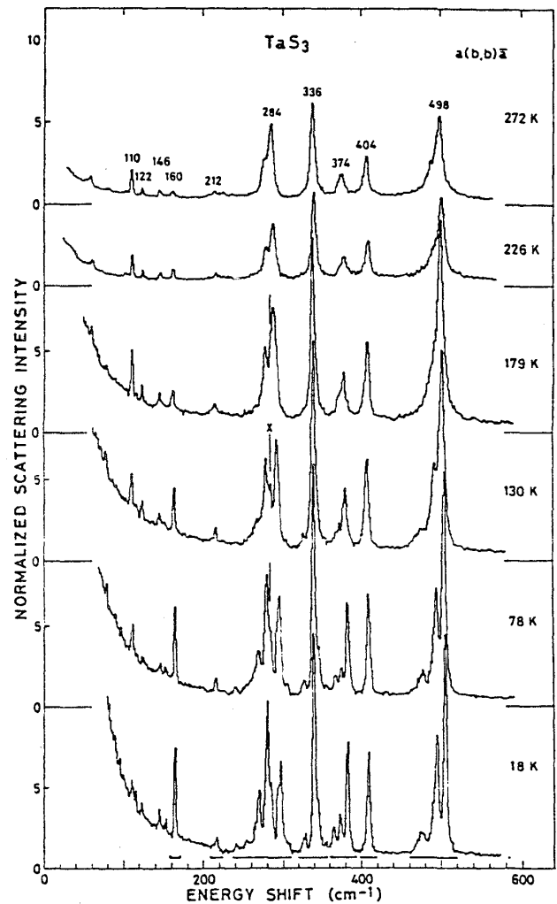
Fig. 1. a(b,b)a配置のラマンスペクトル。
