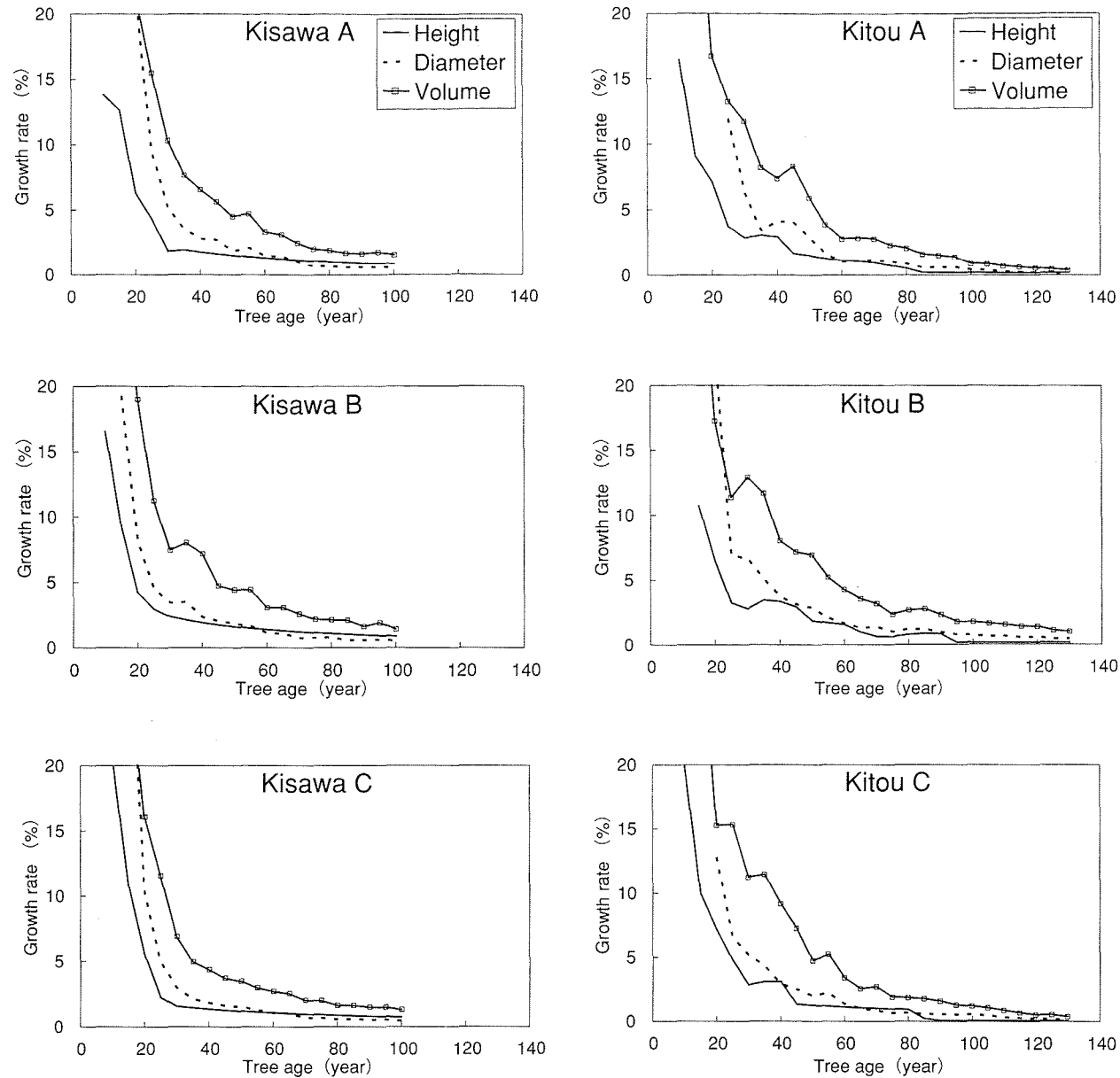
図3 樹高、直径および材積成長率曲線（木沢A～C、木頭A～C） Fig 3 Growth rate curves of height, diameter and volume (Kisawa A-C, Kitou A-C)
