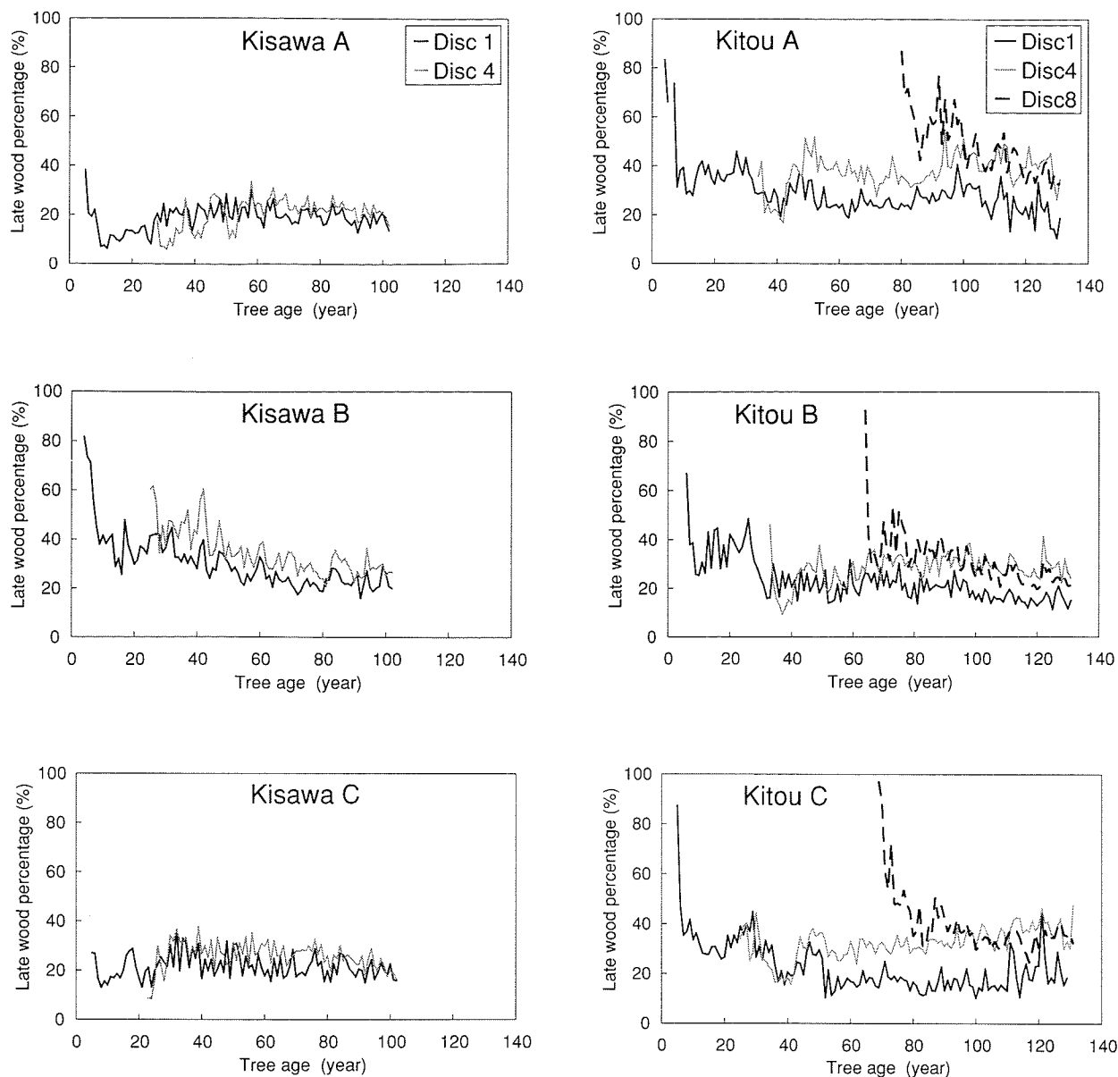
図5 晩材率の水平系列変動 (木沢A~C, 木頭A~C)
