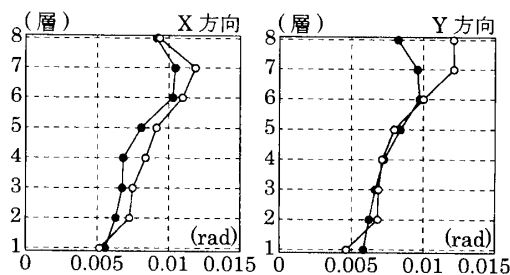
図 5 最大層間変位角 (El Centro NS)
