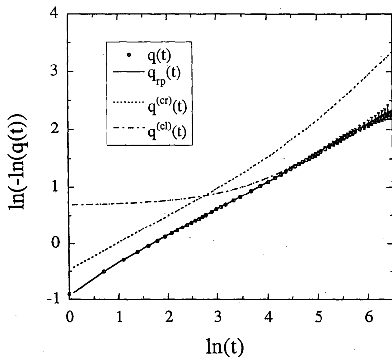
図2： q(t) の Ogielski プロット。データ点は直接シミュレートされた q(t) 。 q^{(\text{cr})}(t) と q^{(\text{cl})}(t) は P(x) の臨界緩和とクラスター緩和ブランチから構築された q(t) で、両者の和が q_{\text{rp}}(t) 。
