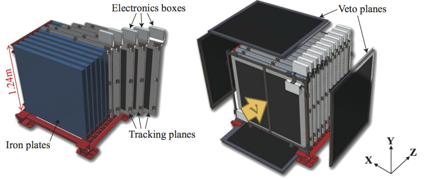
(b) INGRID module
