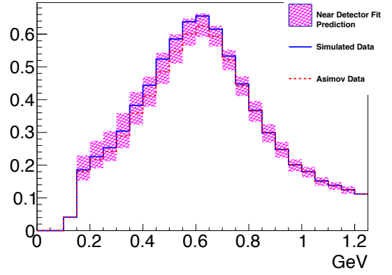
(d) RHC 1Re sample
