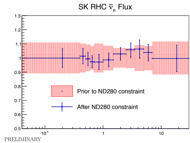
(d) Super-Kamiokande RHC \bar{\nu}_\mu Flux
