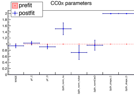
(a) CC0 \pi parameters
