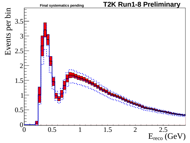
(b) RHC 1R \mu sample
