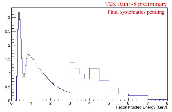
(d) RHC 1R \mu
