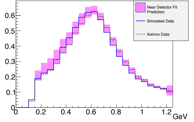
(d) RHC 1Re sample
