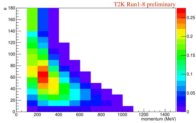
(e) FHC 1Re+1d.e
