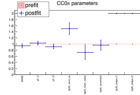
(a) CC 0 \pi parameters
