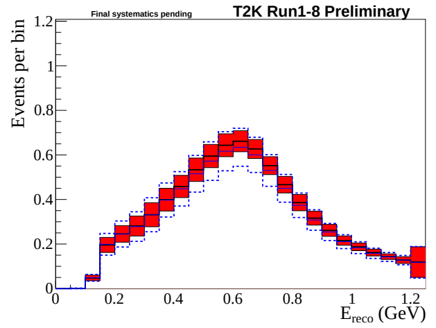
(d) RHC 1Re sample
