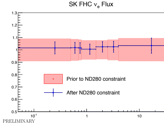
(a) Super-Kamiokande FHC \nu_e flux
