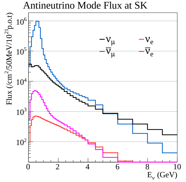
(d) RHC at Super-Kamiokande
