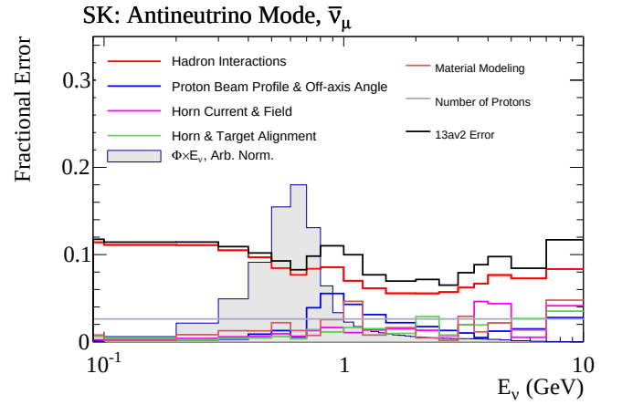
(d) RHC at Super-Kamiokande
