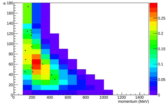
(e) FHC 1Re 1 d.e sample
