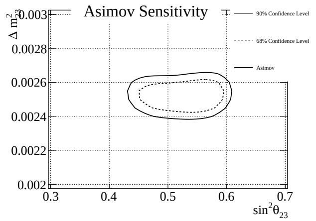
(d) \Delta m^2_{32}
