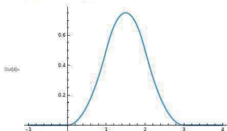
図 8 mathematica での結果
