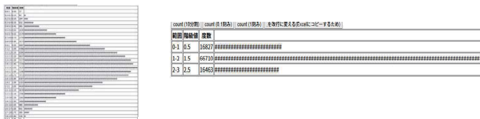
図 7 3 つの一樣乱数の和のヒストグラム表示 (31 分割, 3 分割)
