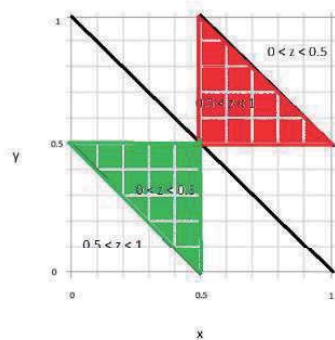
図 2 [0, 1] \times [0, 1] での図示
