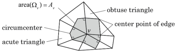
Fig. 2 Area of region D v
