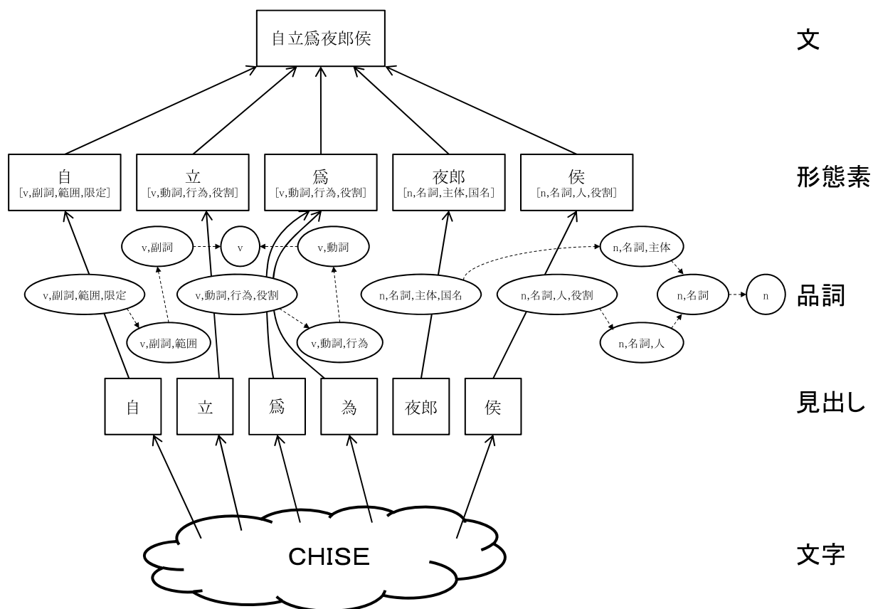
図 3 「自立為夜郎侯」の Linked Data 概念図 Fig. 3 Linked Data around “自立為夜郎侯”.
