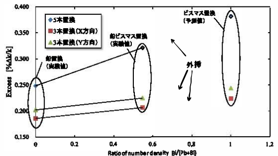
図 2 ビスマスを装荷した炉心の余剰反応度の推定
