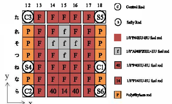
図 1 炉心配置図
