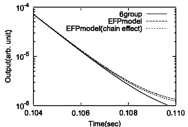
図 1 パルス中性子照射後の挙動変化
