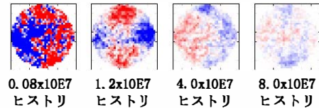
図1. MCNP核分裂中性子源分布の最大値からの差(軸方向位置12/24)
