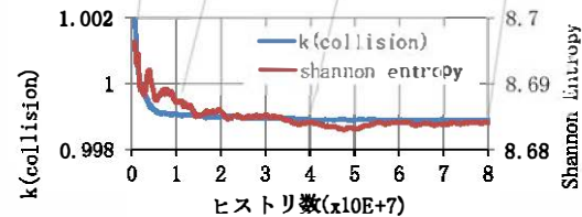
図3. 実効増倍率とShannon Entropyの推移
