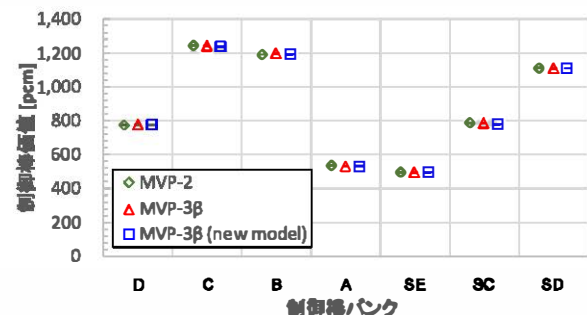
図 2 制御棒価値の測定値との比較
