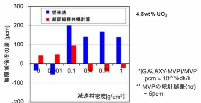
図 1 MVP との無限増倍率の差異 (水密度0~1g/cm 3 )
