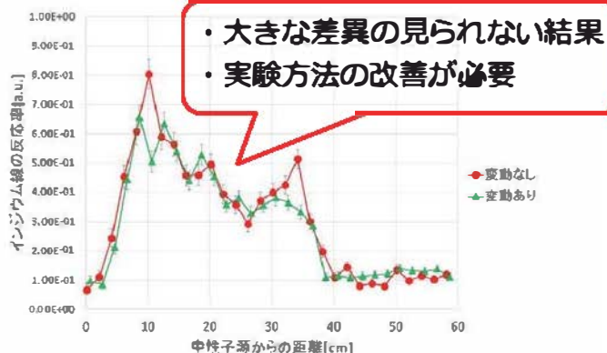
図6. 反応率分布の比較
