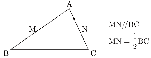
図 7. 中点連結定理
