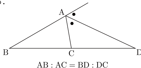
図 13. 外角の二等分線の定理
