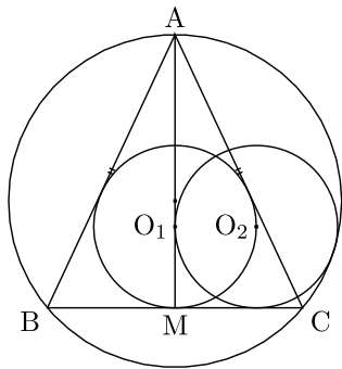
図 17. 福島県田村大元神社の算額
