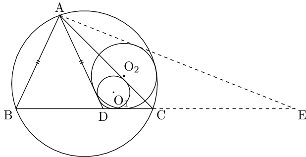
図 15. 宮城県八坂神社の算額
