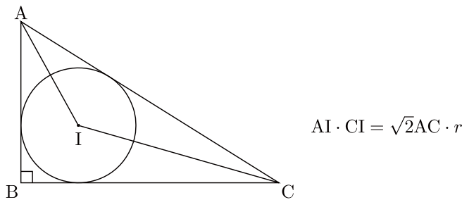
図 11. 福島県熊倉神社の算額
