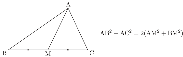
図 10. 中線定理
