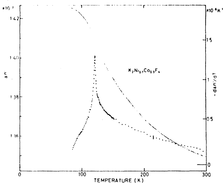
図 1. \text{K}_2\text{Ni}_{0.7}\text{Co}_{0.3}\text{F}_4 の複屈折
