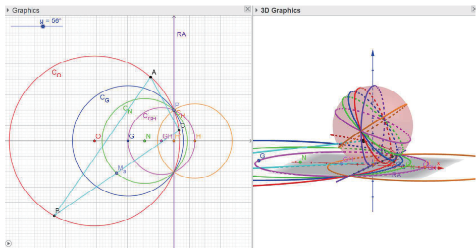
図 2: 鈍角三角形から得られる球面図形.
