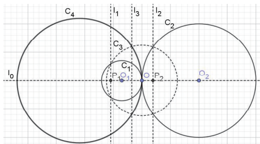
図 6: 接する 2 円の鏡映の軸の作図
