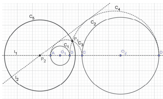
図 3: 離れた 2 円の鏡映の軸の作図
