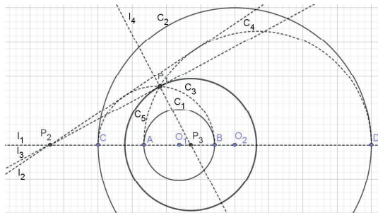
図 5: 包含関係にある 2 円の鏡映の軸の作図
