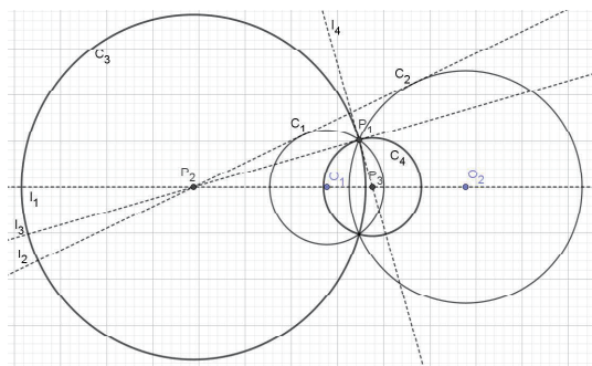
図 4: 交わる 2 円の鏡映の軸の作図
