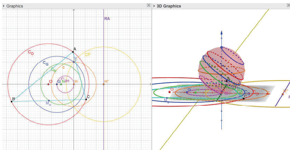
図 1: 鋭角三角形から得られる球面図形.
