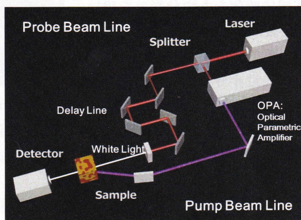
Figure 4 フェムト秒レーザーを光源とする Pump-and-Probe 法による過渡吸収分光装置
