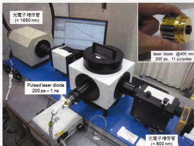
Figure 6 可視・近赤外蛍光分光光度計と時間分解蛍光光源を装着することで、時間分解蛍光寿命測定が可能になるよう設計されている。BHJ素子での励起子拡散－界面電子移動効率の測定に威力を発揮している。
