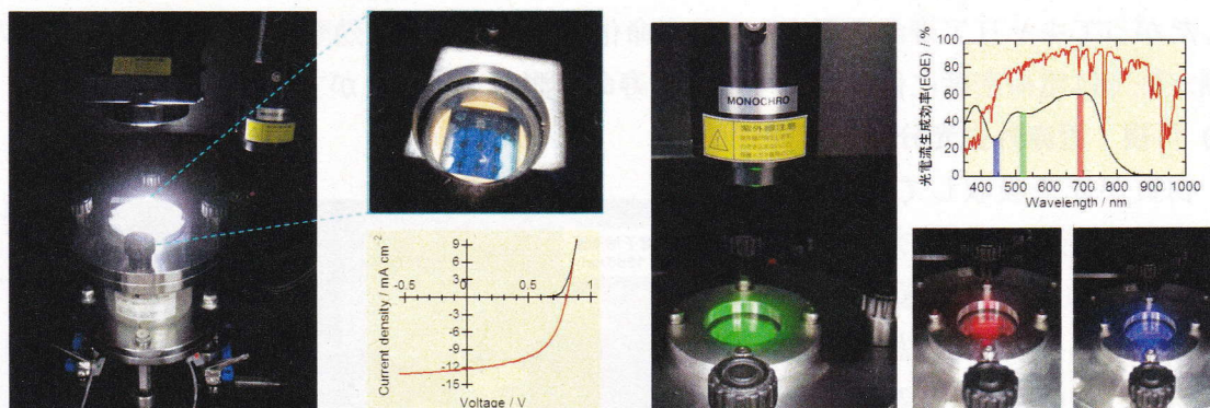
Figure 3 J-V 測定装置 (左)、分光感度測定装置 (右) と得られるデータの例
