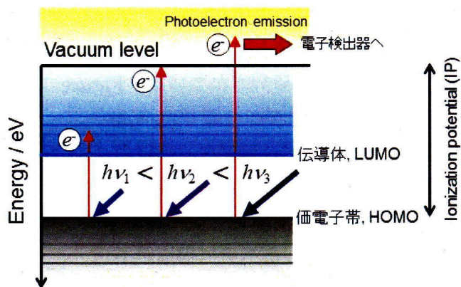
Figure 2 光電子分光法の原理。価電子帯の真空レベルからの深さを測定できる。
