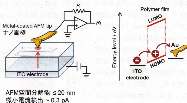
Figure 7 電流計測原子間力顕微鏡(C-AFM)の測定原理図と、電極－材料間のエネルギーレベルの近接によりプローブを流れる電荷
