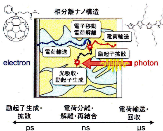
Figure 1 高分子薄膜太陽電池 (BHJ 型素子) における相分離ナノ構造と、その内部で起きる光電変換の素過程
