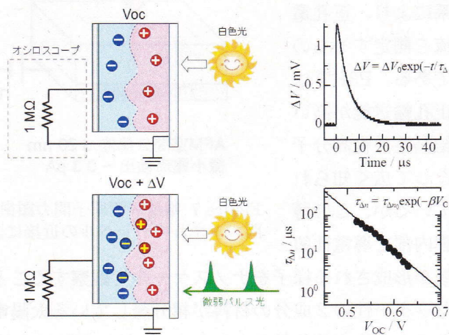
Figure 5 過渡光起電力測定の原理
