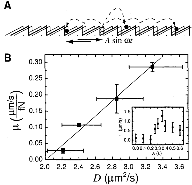
図 1: A Rocking Ratchet の模式図。走査型光ピンセットにより実現した非対称周期ポテンシャルを sine 型に揺るとトラップされたビーズの拡散運動に方向性が生じる。 B 光学 rocking ratchet における拡散係数と移動度の関係。ポテンシャルを揺らした状態で拡散係数と移動度をそれぞれ測定し、両者の関係をプロットした。左下から振幅 A = 0L , 0.20L , 0.26L , 0.40L でのデータを表す。ただし L はポテンシャル周期 ( 2.5 \mu\text{m} )。Inset: 各振幅 A における、無負荷でのビーズの平均速度。A の右方向を正にとってある。
