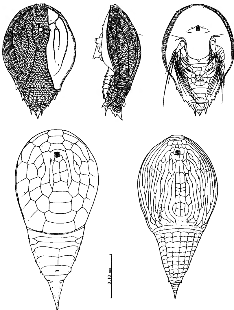
第1図 田辺湾で発見された3種のノープリウスy. 上段は同じ個体の背面、側面、腹面を示す。 (Itô 1986 による)
