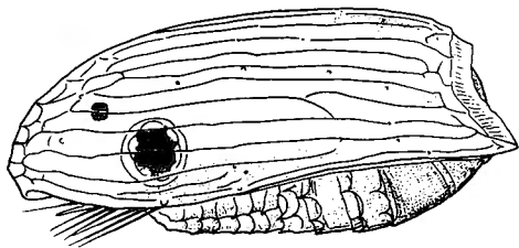
第3図 bending behavior を示すキプリス y.
