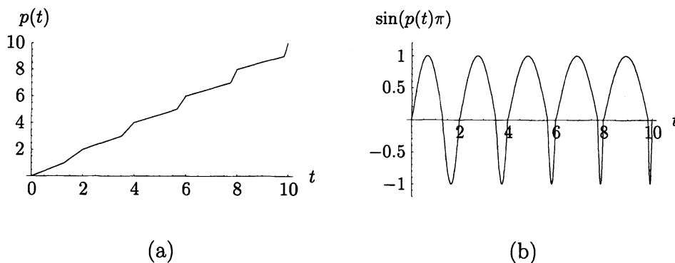
(a) r = 0.7 の場合の p(t) のグラフ; (b) r = 0.7 の場合の \sin(p(t)\pi) のグラフ
