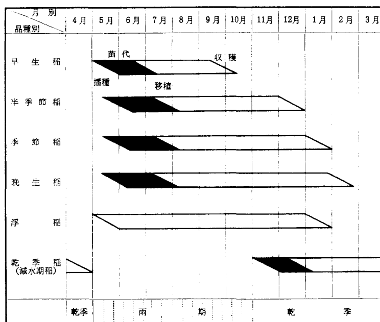
図-1 水稻の品種分類別栽培期間
