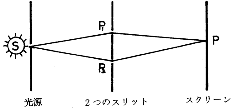
図 1. Young の実験
