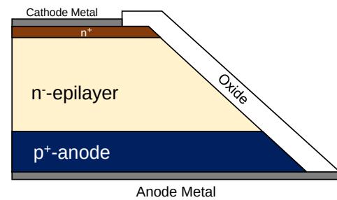
(d) Positive Bevel Termination
