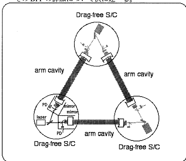
図1 DECIGO 構成図
