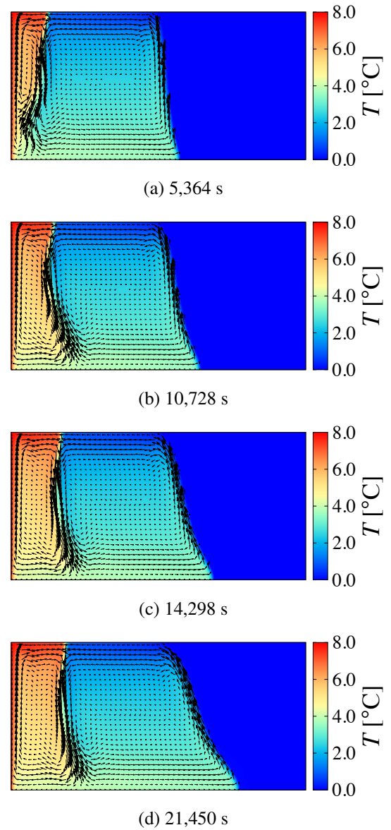
図-14 各時刻における温度分布および流速ベクトル
