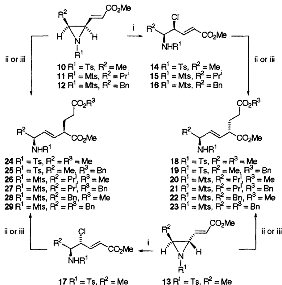
Scheme 3. Reagents: i, 4 M HCl/1,4-dioxane; ii, \text{IZn(CN)CuCH}_2\text{CH}_2\text{CO}_2\text{Me}\cdot 2\text{LiCl} ; iii, \text{IZn(CN)CuCH}_2\text{CH}_2\text{CO}_2\text{Bn}\cdot 2\text{LiCl} .
