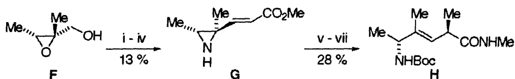
Scheme 2. Reagents: i, DMSO, (COCl) 2 , Et 3 N; ii, Ph 3 P=CHCO 2 Me; iii, NaN 3 , NH 4 Cl, iv, Ph 3 P; v, Boc 2 O, Et 3 N; vi, Me 2 Zn·2LiCl, CuCN; vii, MeNH 2 , NaCN.
