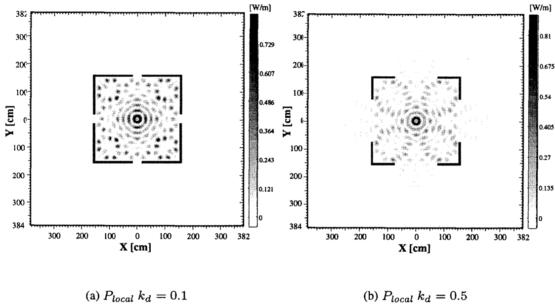
図 3.9 窓の大きさと平面波電力密度分布 P_{local} の関係。(a) は平均散逸確率が k_d = 0.1 の状況で、外部へのエネルギー流出は殆ど見られない。(b) は平均散逸確率が k_d = 0.5 の状況で、エネルギー流出が確認される。
