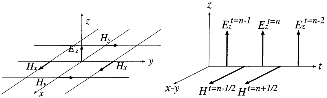
(a) FDTD 法：空間差分概念図
