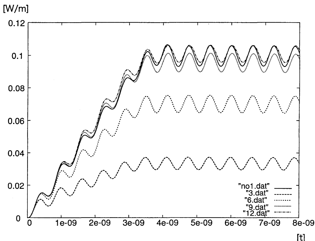
図 3.10 吸収散乱体と波源の距離（吸収散乱体なし、および距離 3cm, 6cm, 9cm, 12cm）と平均電力密度の関係：実線は吸収散乱体なしのデータ、 x.dat は吸収散乱体と波源との距離が x のデータである。波源の出力は 0.6[W] 周波数 800MHz
