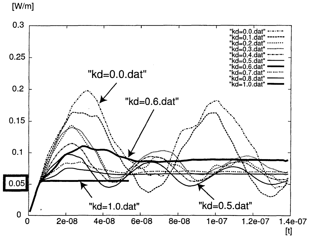
図 3.8 数値実験から求めた平均電力密度 \langle P \rangle の時間発展。平均散逸確率を変数とした。 k_d = 0.6 でエネルギーバランス方程式とおおよそ一致。 k_d = 1.0 は窓がない時。
