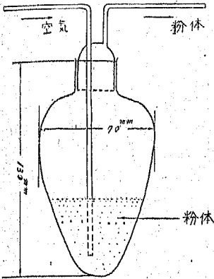
第3圖 送風管の形狀
