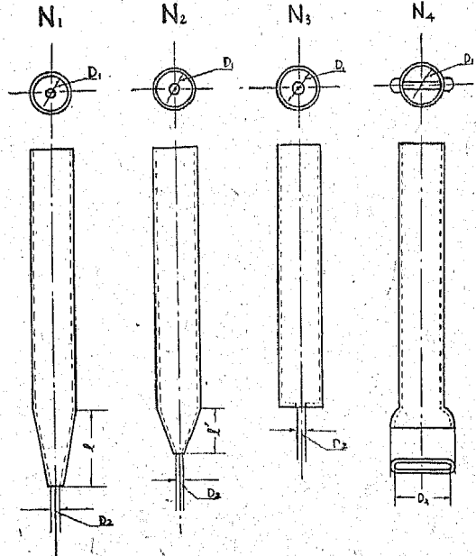
第5圖 撒粉口の形狀
