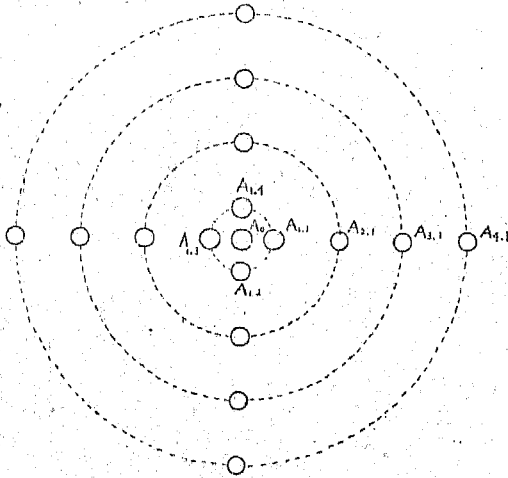
第6図 受皿の配置図
