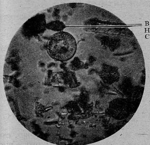
第10図 BHC と担体の混合状態の顕微鏡写真 (780 X)
