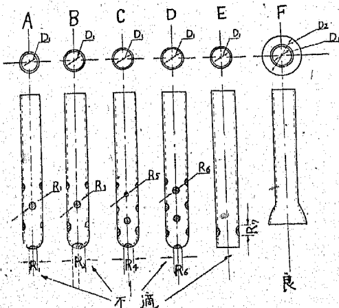
第4圖 撒粉室
