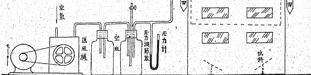
第8図 人工雨に対する固着度の 測定装置
