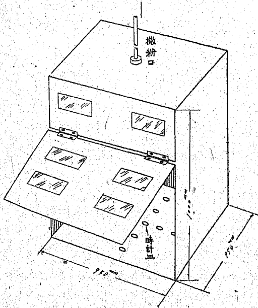
第4圖 撒粉室
