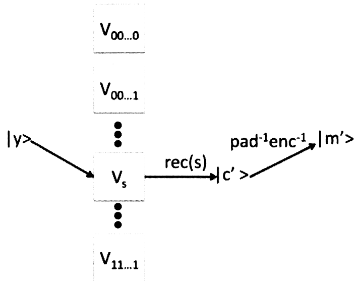
図 2: 復号器の過程
