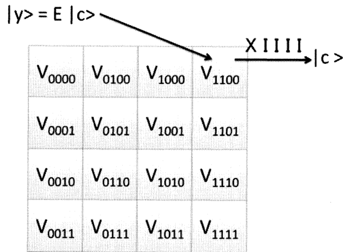
図 3: 5量子ビット符号の復号過程
