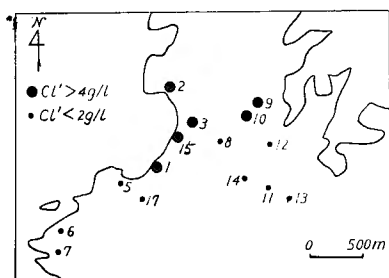
Fig. 7. Distribution of hot springs in Shirahama Spä.
