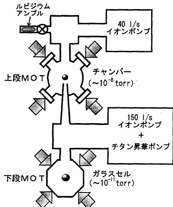
図3. 二重磁気光学トラップ
