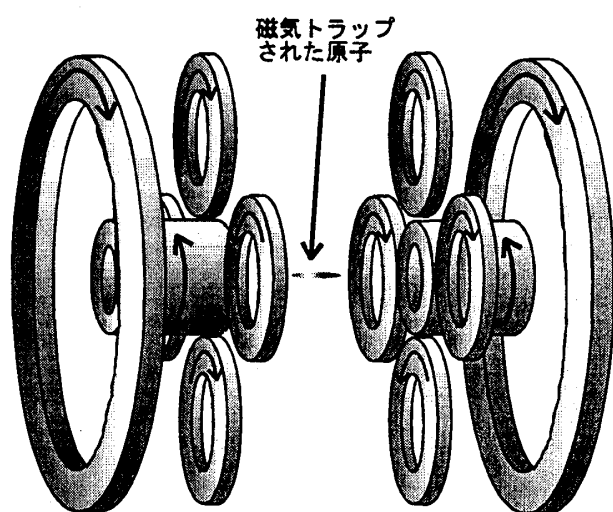
図4. クローバーリーフコイル
