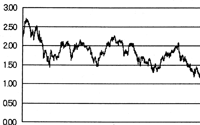
Fig.1.1: NIKKEI 225 from Jan.1991 to Sep.2001
