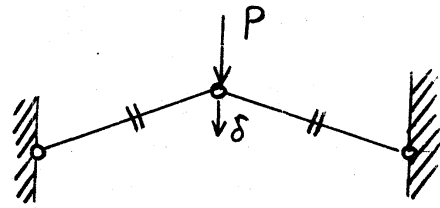
図-2 3-ヒンジ骨組
