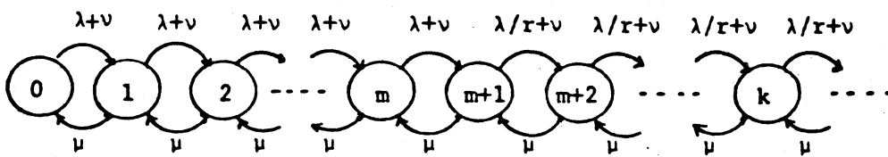
図8 Level 3 の配送法の状態遷移率図
