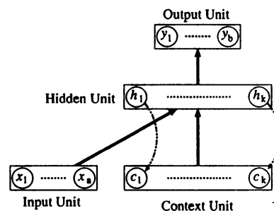
図 1: 単純回帰ネットワーク
